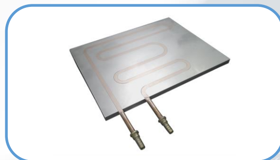
冷板式液冷—埋管工艺
